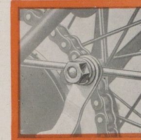
Gabel-Gelenk an der Hinterrad-Bremse
