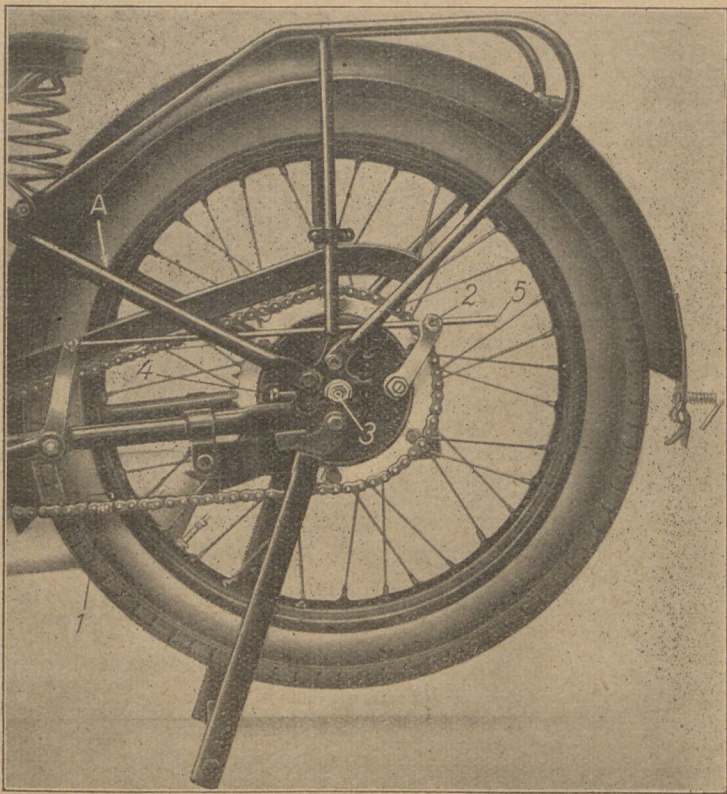
(Bild 14) Hinterrad
