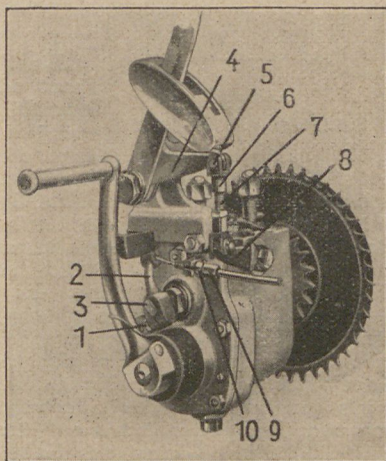
(Bild 9) Zündapp-Dreigang-Getriebe
