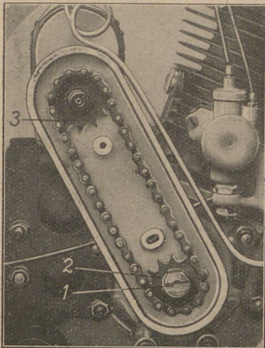
(Bild 6) Nachstellen der Zündung
