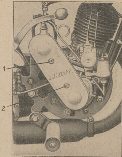
(Bild 5) Nachstellen der Zündung
