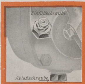
Getriebe
