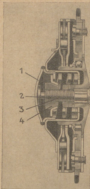
(Bild 10) Schnitt durch die Kupplung
