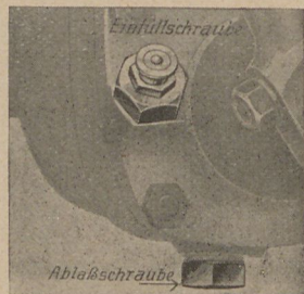
(Bild 8) Getriebe-Schmierung
