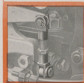
Gabel-Gelenke an der Getriebe-Schaltung
