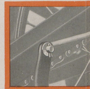
Gabel-Gelenk am Fuß-Bremshebel
