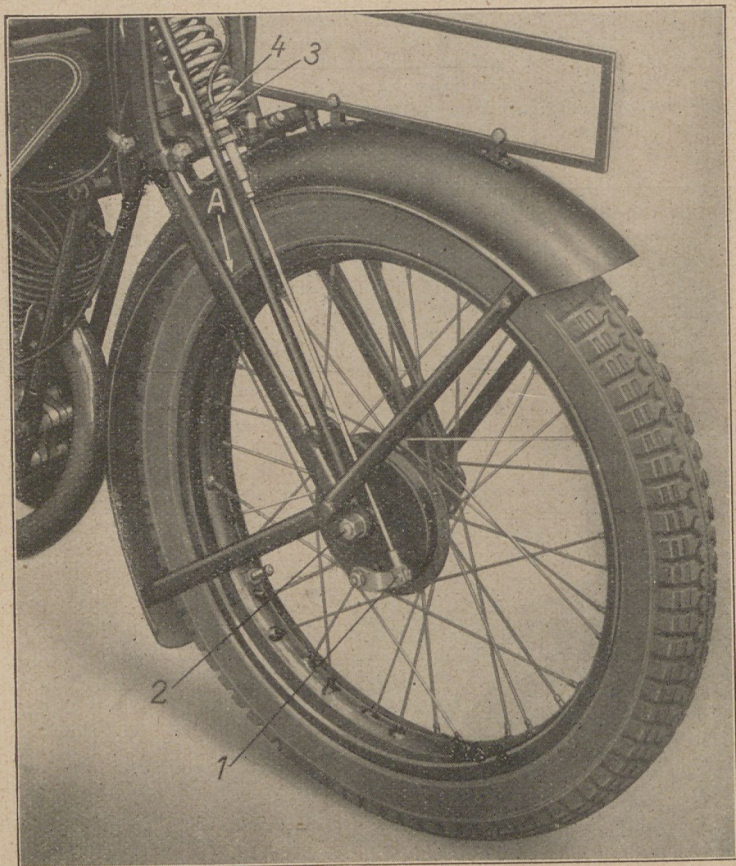
(Bild 13) Vorderrad
